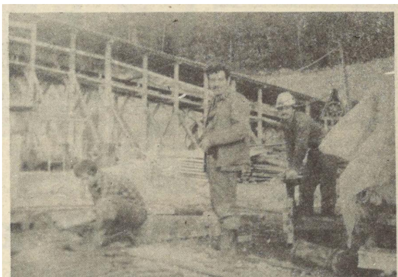
V DVEH LETIH 210 MILIJONOV DINARJEV ZA NAHAJALIŠČE LIGNITA V GLOBOKEM — Raziskovalna vrtanja so v polnem teku. Trenutno nadaljujejo z izkopom izvažalnega vpadnika, vendar jim dotok vode in vdiranje mulja povzročata precejšnje težave. Zračilni jašek je do 185 metrov globine presekala tri krovne sloje lignita, debeline 25 do 80 cm. Na območju rudnika je deset milijonov ton premogovnih zalog. Lignit je podoben velenjskemu, vendar vsebuje manj žvepla. Rudnik bodo odprli 1987. Na leto bodo izkopali od 250 tisoč do 500 tisoč ton premoga. (Foto: Jožica Teppey)
